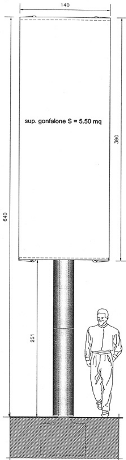
prospetto
